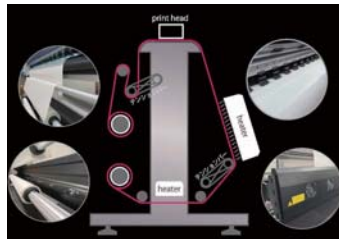
【転写紙の流れ】
